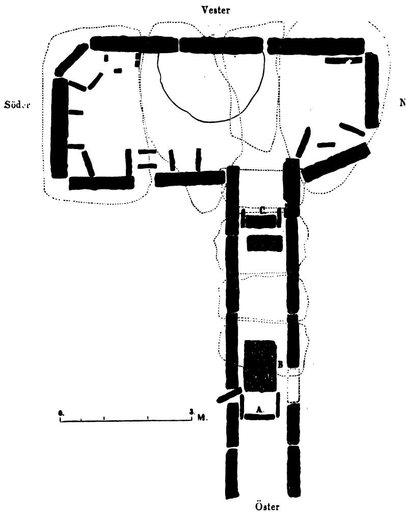
97. Plan af gånggriften fig. 95 vid Karleby i Västergötland. A den yttre tröskel och dörrposterna; B dörren; C den inre tröskeln och dörrposterna.
