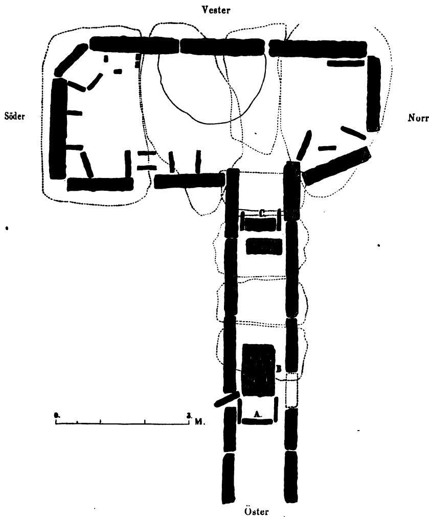
8. Plan af en graf från stenåldern (gånggrift) i Vestergötland.
