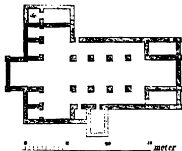
434. Plan af Alvastra klosterkyrka.
