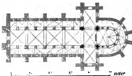
436. Plan af Varnhems klosterkyrka.
