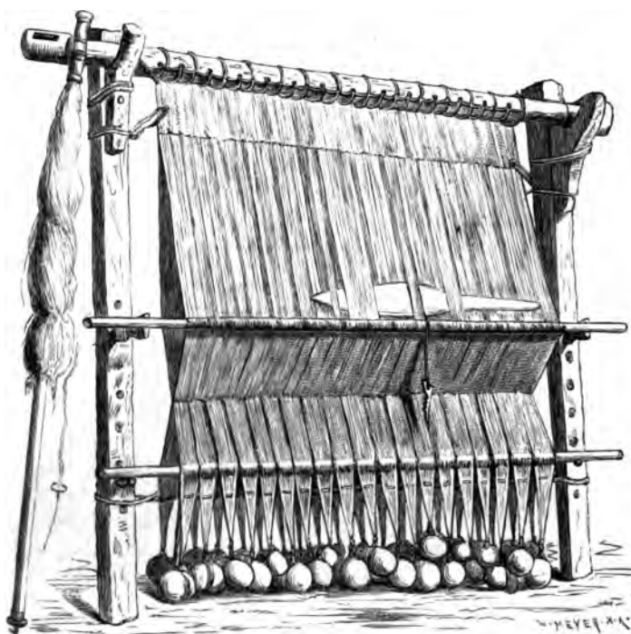
382. Väfstol från Färöarna. 1 / 10 .
