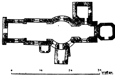
472. Plan af Solna kyrka 2 .
