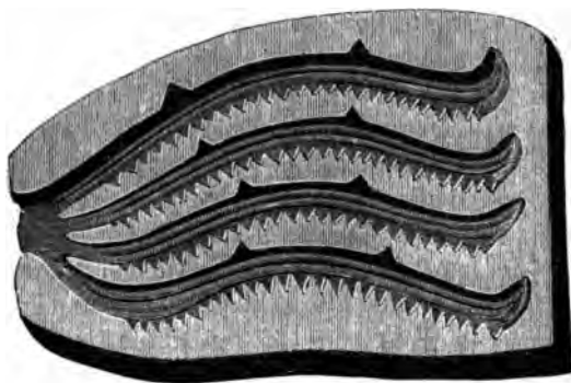
209. Form af sten för gjutning af fyra sådana bronssågar som fig. 210. Skåne. \frac{1}{2} .
