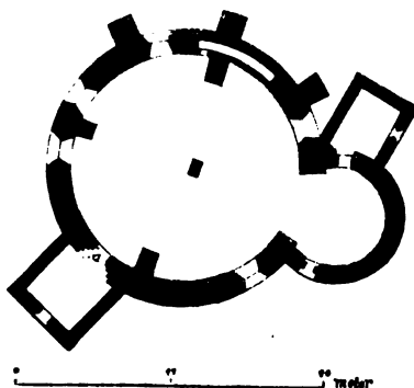
465. Plan af Hagby kyrka.
